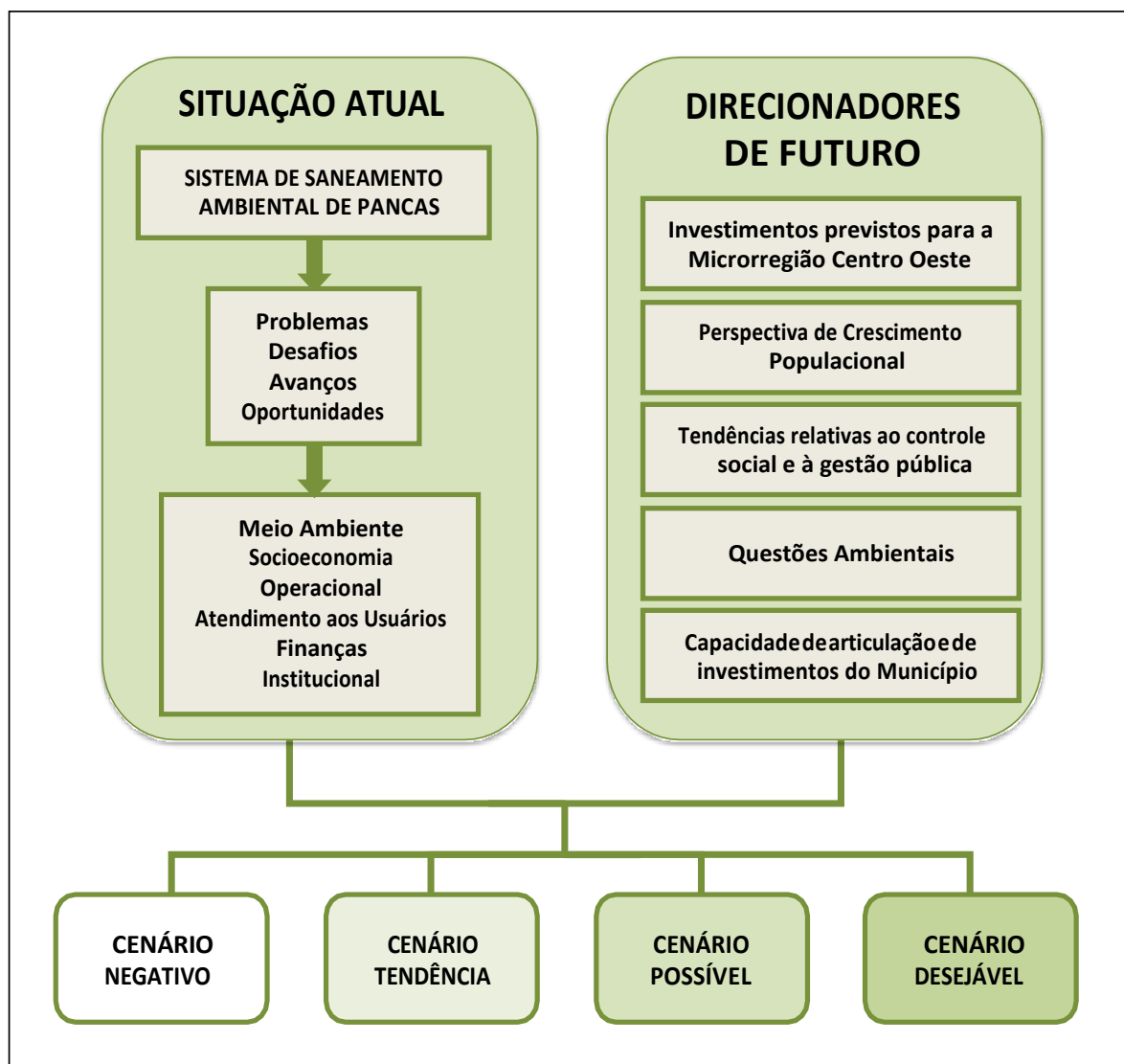
Figura 4-1 - Esquema metodológico.
