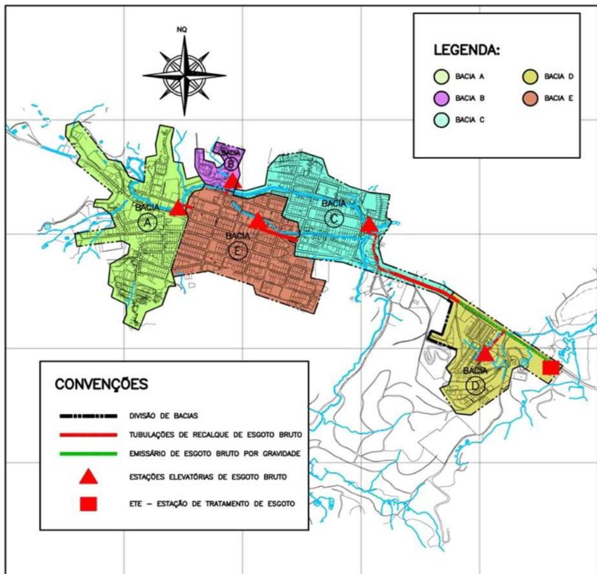
Figura 3-20: Planta esquemática do SES em Pancas Sede.
